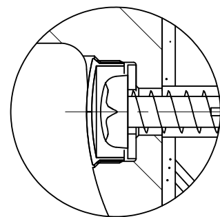
④ねじ隠しキャップ部詳細 (S=1/1)
